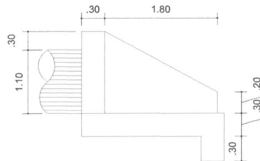
VISTA LATERAL
