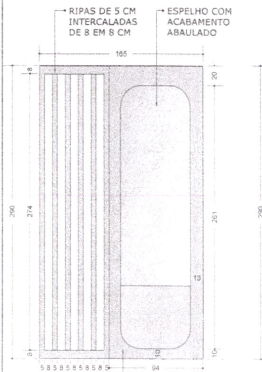
VISTA A | 1:25
