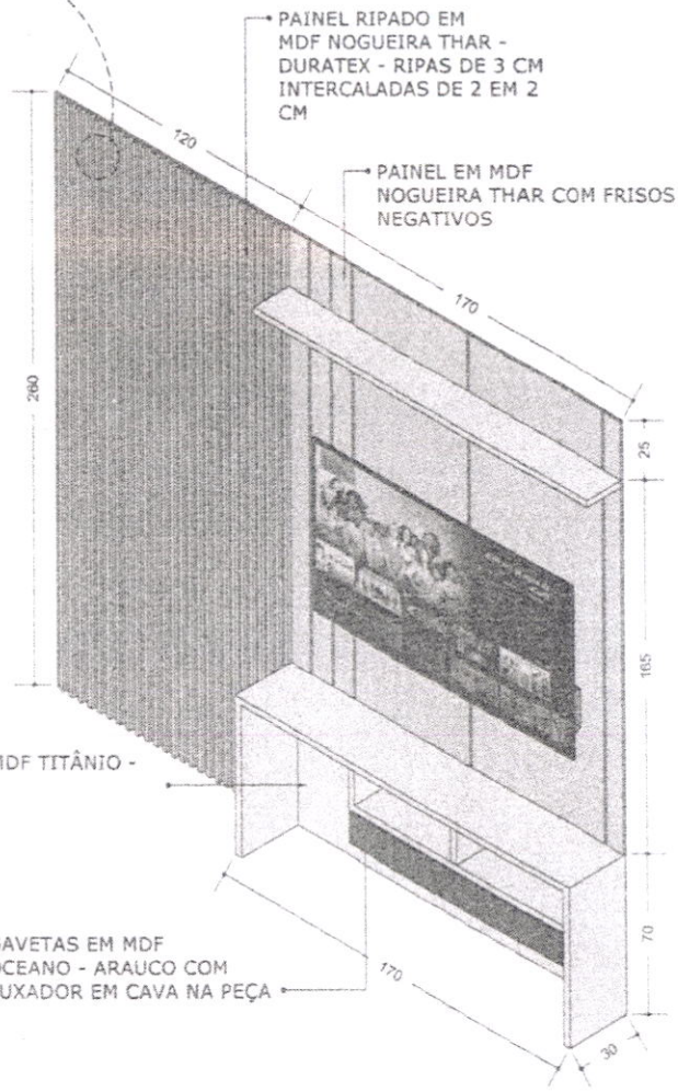
PERSPECTIVA | 1:20
