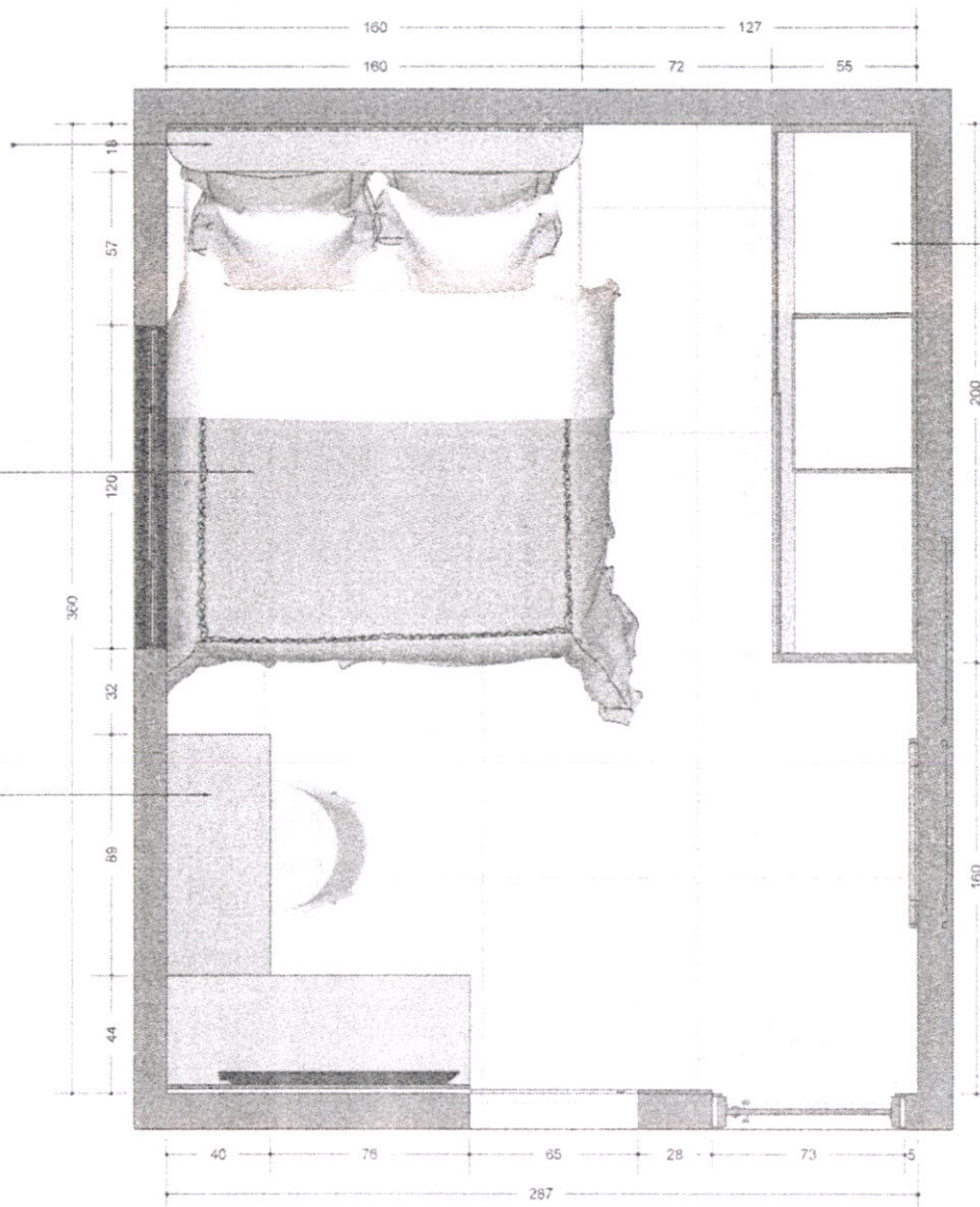
10 PLANTA BAIXA - QUARTO 02 ESCALA: 1/20
