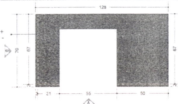
PLANTA BAIXA | 1:15
