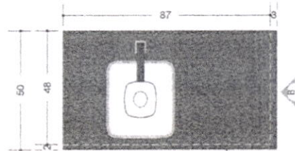
PLANTA BAIXA | 1:15
