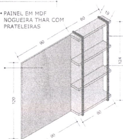
PERSPECTIVA | 1:20
