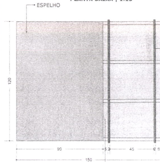
VISTA A | 1:15
