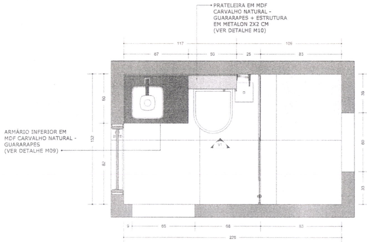
09 PLANTA BAIXA - BANHO SOCIAL ESCALA: 1/15
