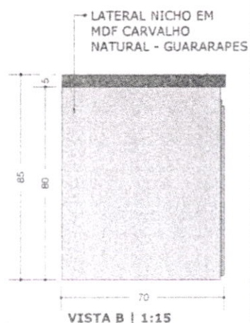
VISTA B | 1:15
