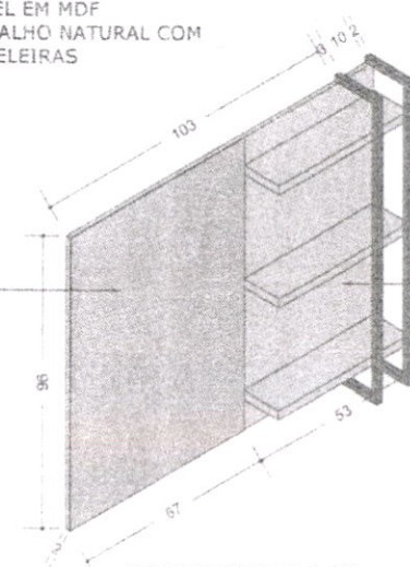
PERSPECTIVA | 1:15
