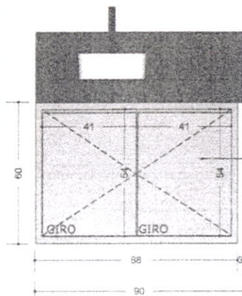
VISTA A | 1:15
