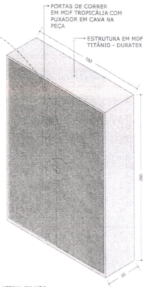
PERSPECTIVA | 1:20
