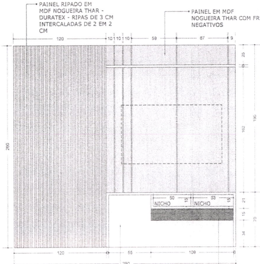
VISTA A | 1:20
