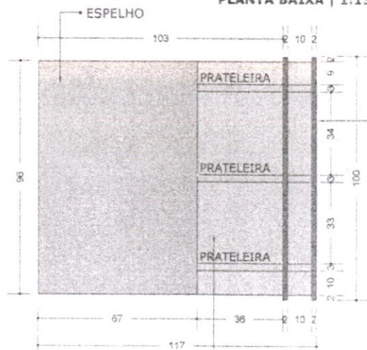
VISTA A | 1:15
