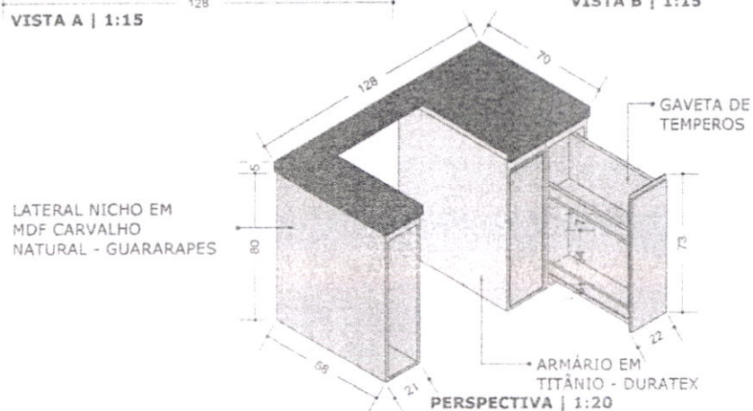
PERSPECTIVA | 1:20
