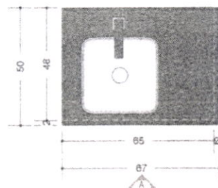
PLANTA BAIXA | 1:15
