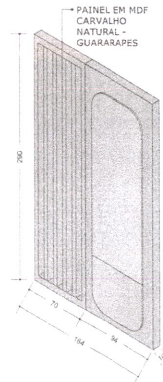
PERSPECTIVA | 1:25
