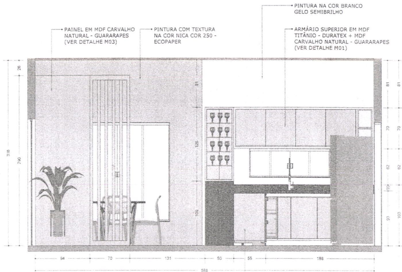
02 VISTA A ESCALA: 1/25
