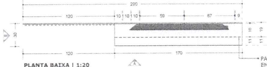
PLANTA BAIXA | 1:20
