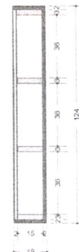
VISTA B | 1:15
