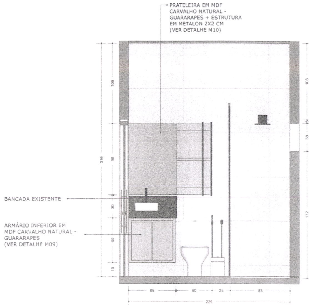
10 VISTA 01 - BANHO 01 ESCALA: 1/20
