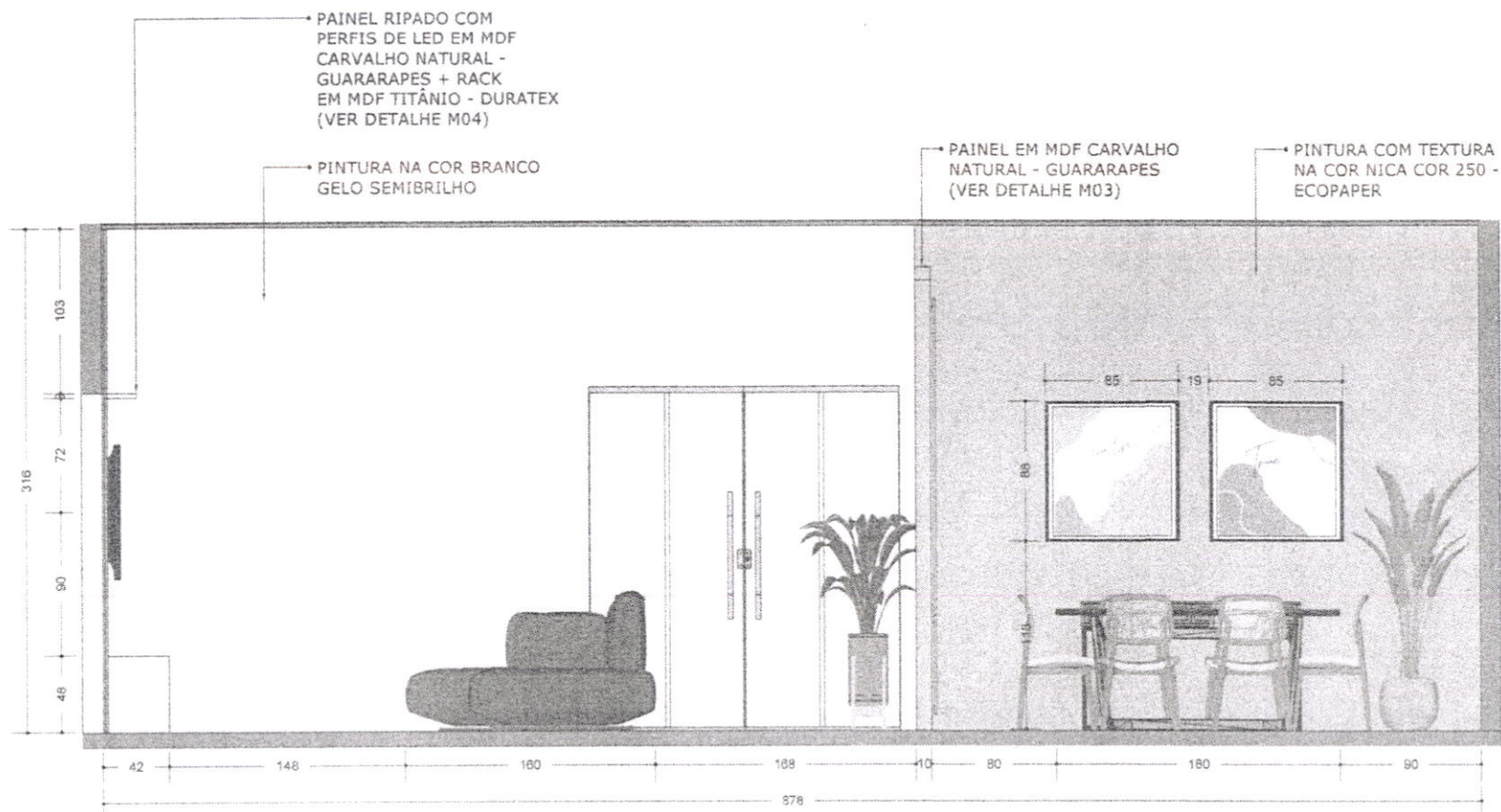
02 VISTA B ESCALA: 1/30
