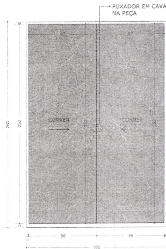
VISTA A | 1:20
