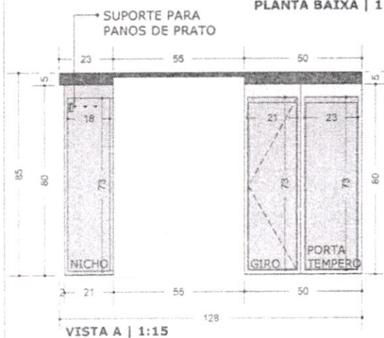
VISTA A | 1:15
