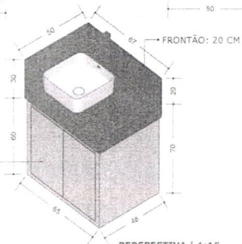
PERSPECTIVA | 1:15
