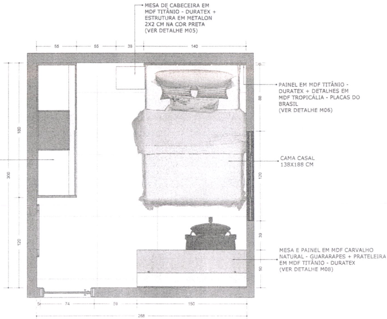
08 PLANTA BAIXA - QUARTO 01 ESCALA: 1/20
