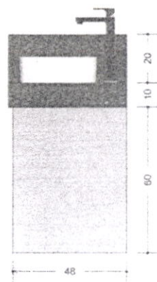
VISTA B | 1:15
