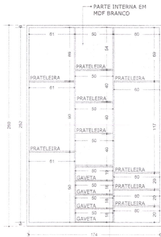
VISTA A - INTERNA | 1:20
